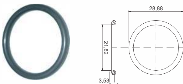
ANEL O'RING COMANDO DO GARFO
