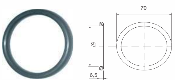
ANEL O'RING DA TAMPA DA CAMISA DO PISTÃO
