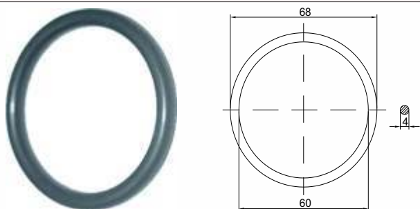
ANEL O'RING EM CORDÃO DE P.U. CORRUGADO
