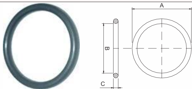
ANEL O'RING VÁLVULA ISOBÁRICA
