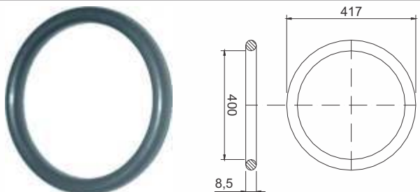
ANEL O'RING DOSADOR DE LÚPULO
