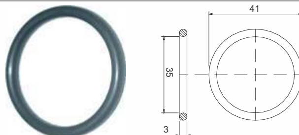
ANEL O'RING DA TAMPA DO PNEUMÁTICO
