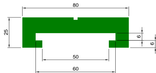
PERFIL TRP DA ENTRADA DA REGRAVADORA
