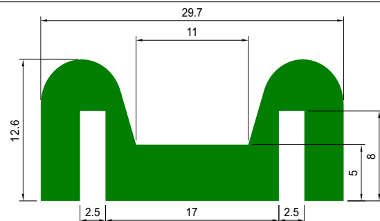
PERFIL M CLIP
