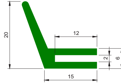
PERFIL L - DUPLO
