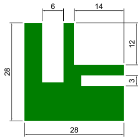
PERFIL INFERIOR DO TRP CURVA ECX
