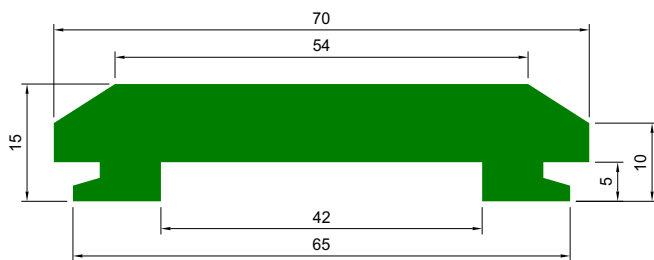
PERFIL RÉGUA DO SNIFF
