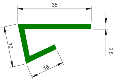
PERFIL L - COM GRAU
