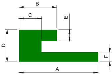
PERFIL L - COM ABA
